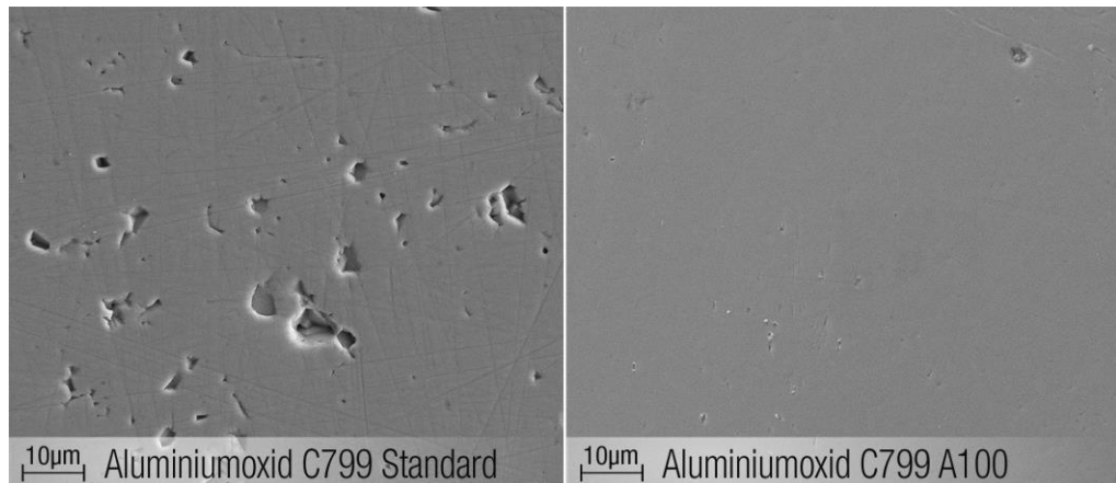
Bild 2: Vergleich der keramischen Struktur, polierte Oberflächen \text{Al}_2\text{O}_3 C799 Standard / \text{Al}_2\text{O}_3 C799 A100
